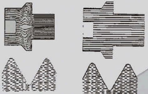
(A)鍛造滾牙螺絲具連續性鍛流線 (B)切創螺絲之鍛流線
