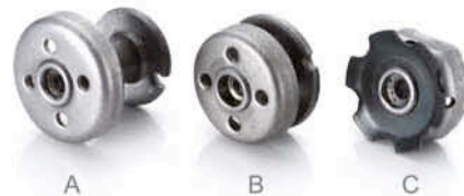
Model : SHL 14 Expander for fork stem Size : M6*10 · 18 · 30mm
