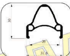
20" 24" 26" 27.5" RIM 20" (406) WD RIM
