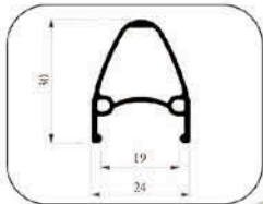
20" 24" 26" 27.5" RIM 20" (406) WD RIM
