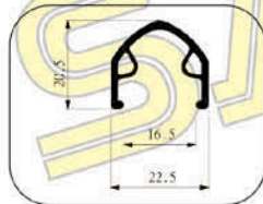
16" 305 RIM 24" (540), 700C RIM
